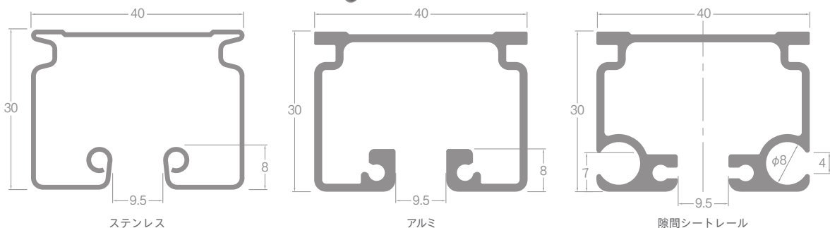
レール断面図 (単位: mm)
