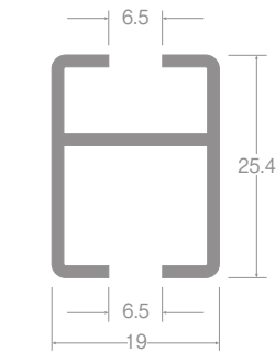
レール断面図 (単位: mm)
